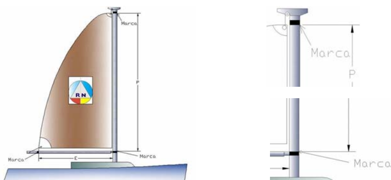
Imagen 16. Grátil de mayor, P
