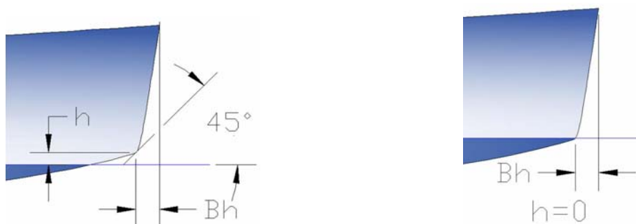
Imagen 10. Altura del lanzamiento de proa, "h"
