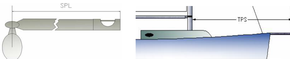
Imagen 23. Longitud del tangón y botalón, SPL, TPS
