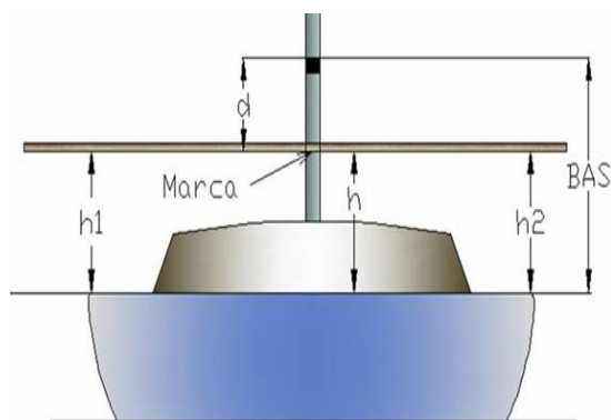
Imagen 20. Altura de botavara, BAS
