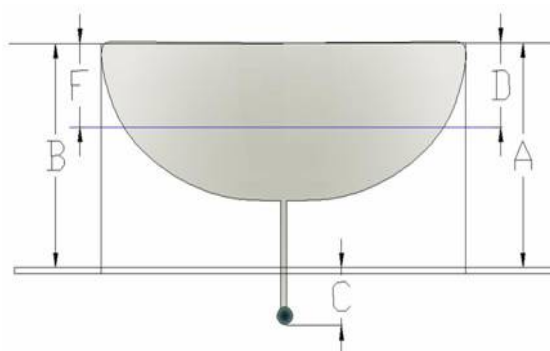
Imagen 8. Cálculo calado
